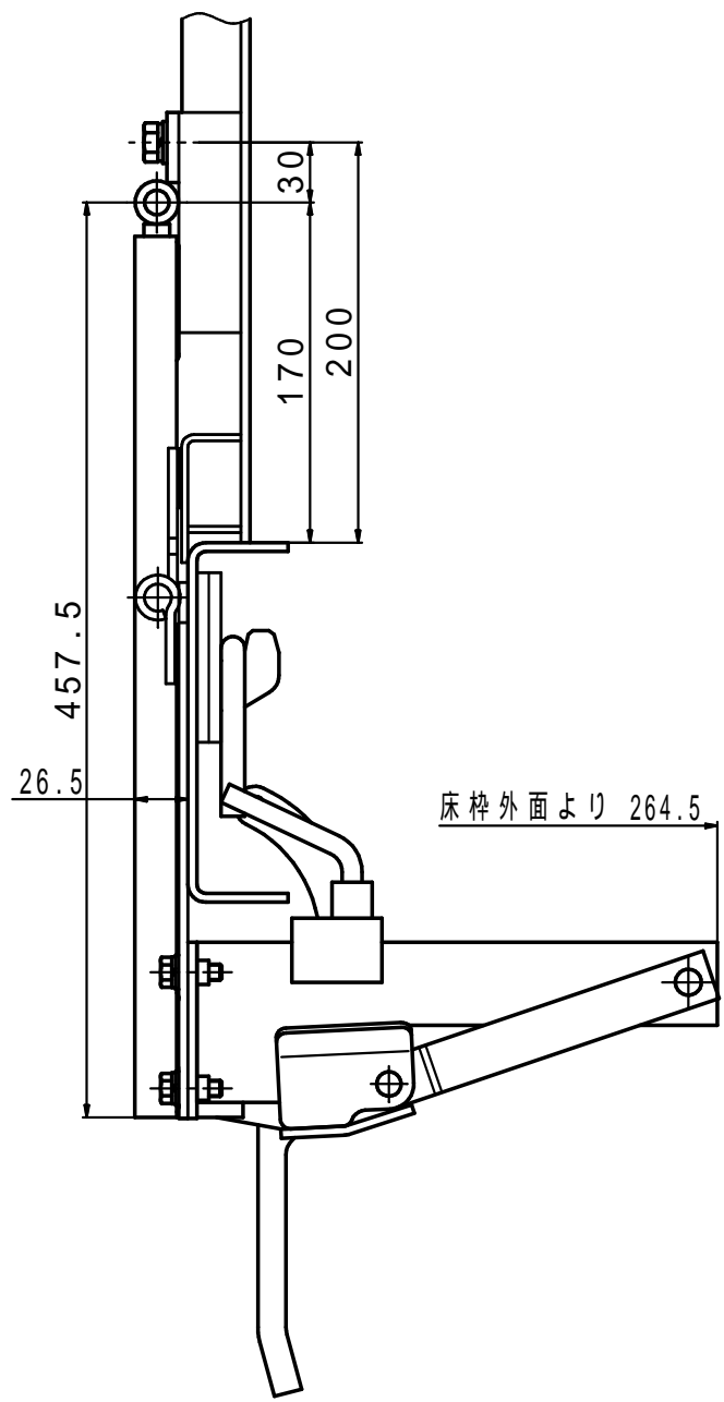
名称 セイコークットII型 - M(トレー用) 外観図
